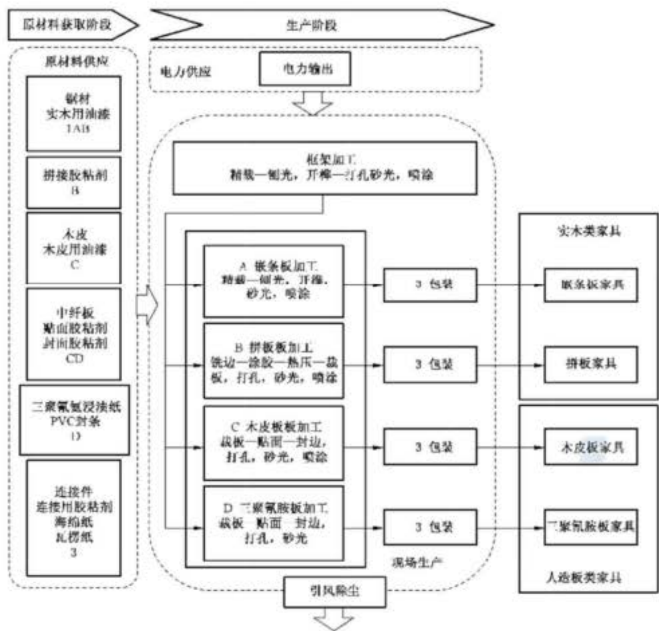
图 B.1 木制家具产品系统边界
