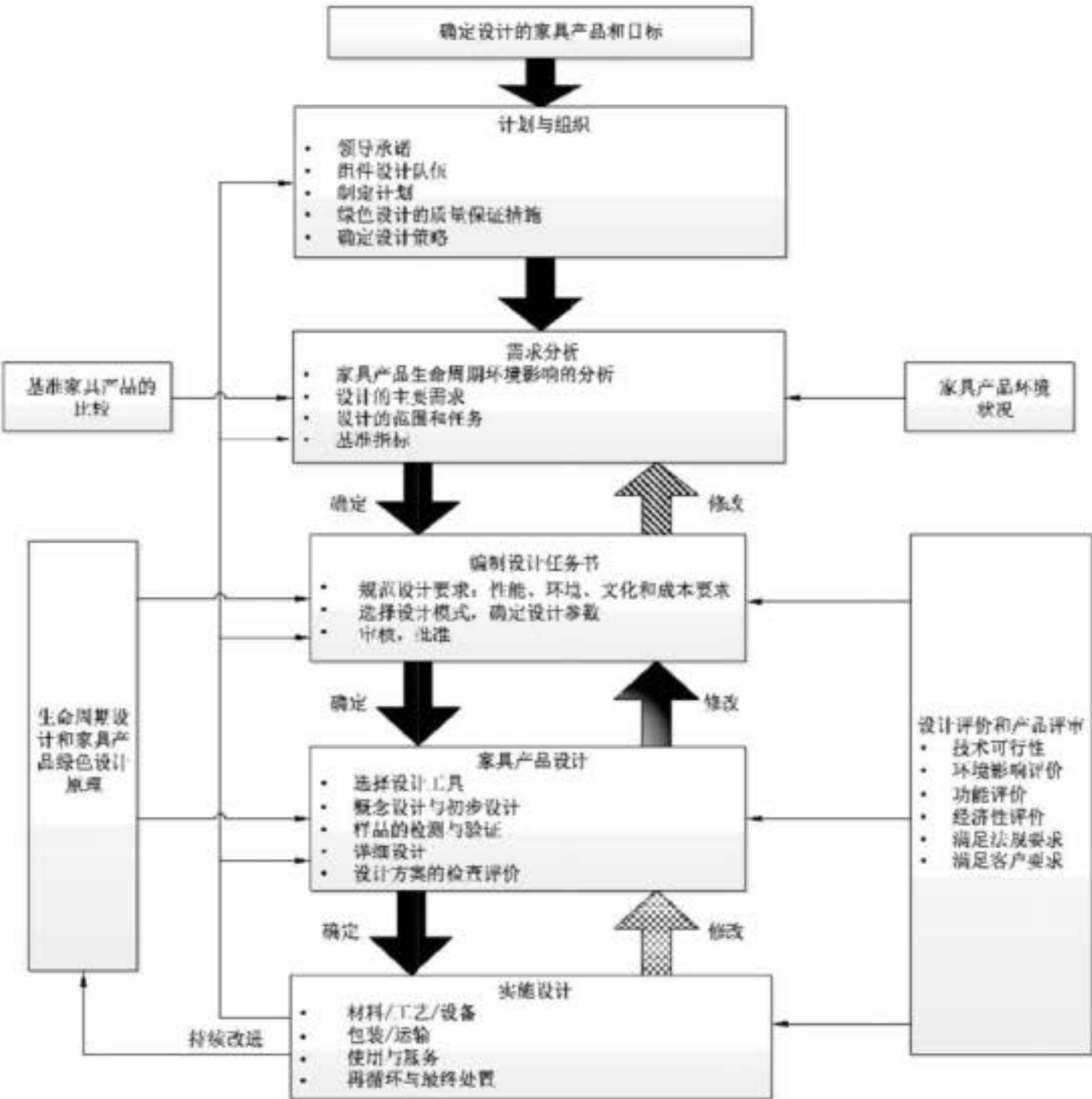
图 1 产品绿色设计过程示意图
